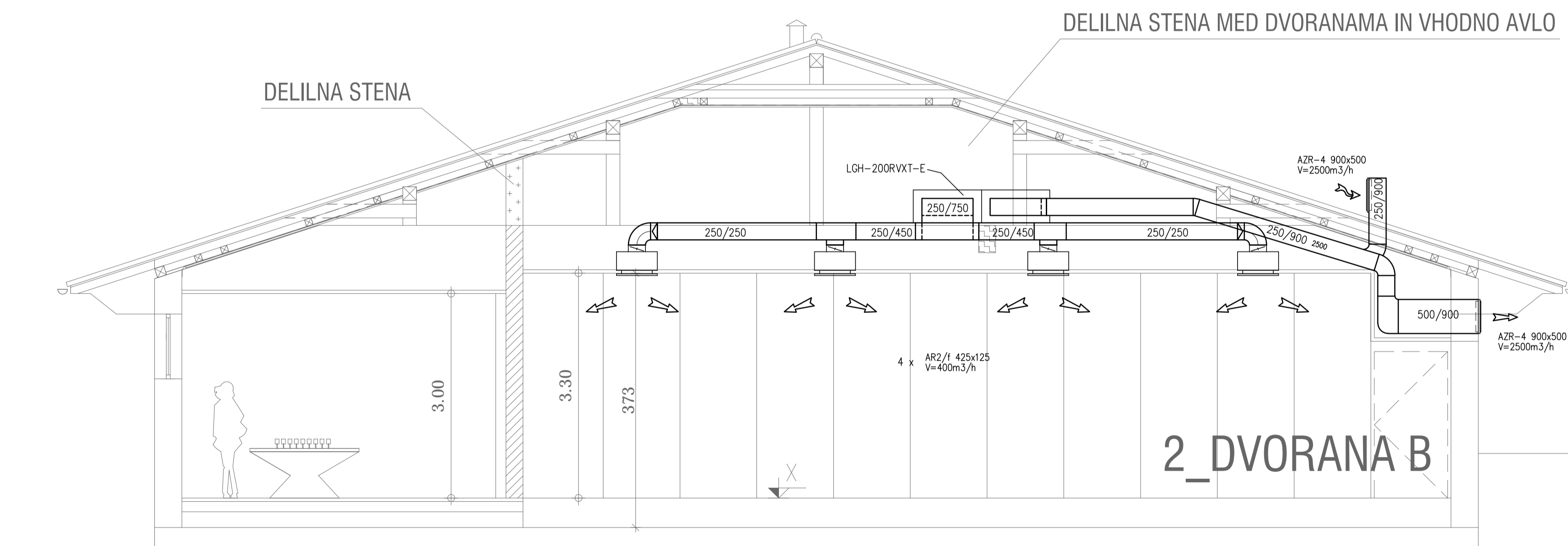
PREREZ A-A
