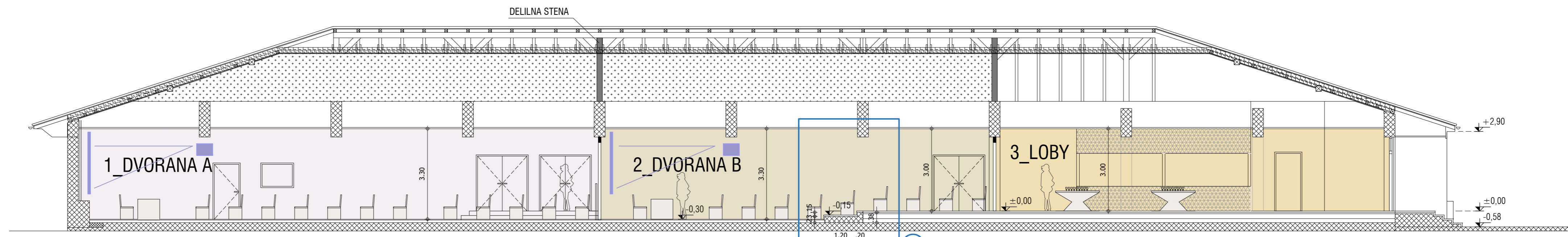
PREREZ A-A
