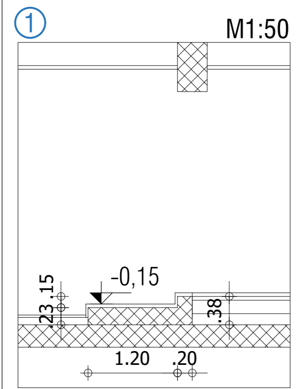
PREREZ B-B
